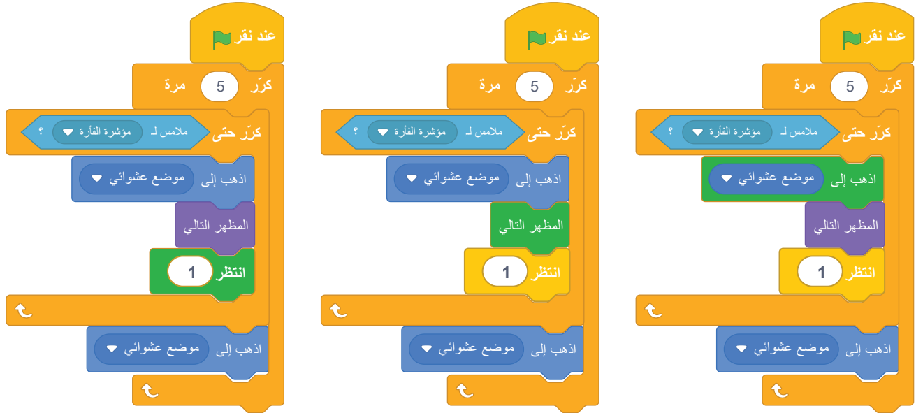
الشكل (3-5): تنفيذ لبّات الحلقة الداخلية.
